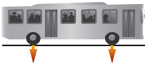
Σχήμα 3.5 Ομοιόμορφη και ανομοιόμορφη επί των αξόνων φόρτωση.
