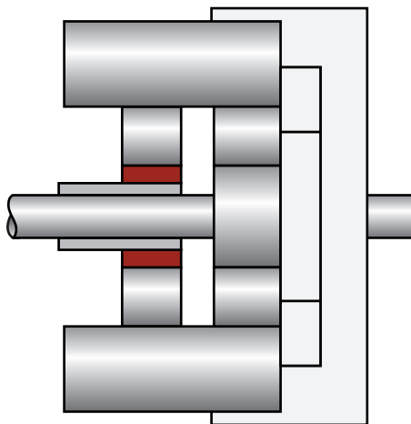
Σχήμα 2.15 Μειωτήρας.
