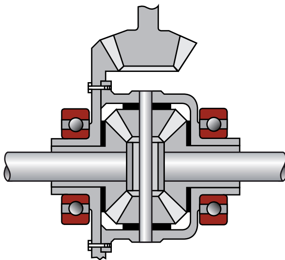
Σχήμα 2.14 Διαφορικό.
