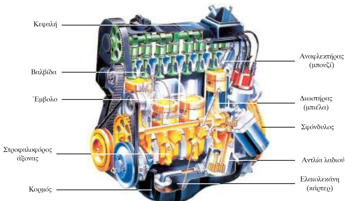
Σχ. 2 Τομή τετρακύλινδρου βενζινοκινητήρα.
